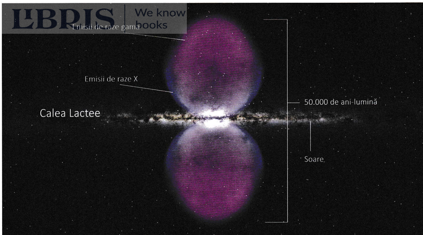
Fig. 1-3. Imagine a galaxiei Căii Lactee care prezintă niște bule uriașe de raze gama ce se întind pe 50.000 de ani-lumină, adică aproape jumătate din diametrul galaxiei. Detectate de telescopul Fermi (culoarea magenta) și observate anterior în raze X de către ROSAT (culoarea albastră). Centrul de Zbor Spațial Goddard al NASA.
